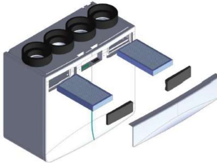
Рис. 5 – Заміна фільтрів
